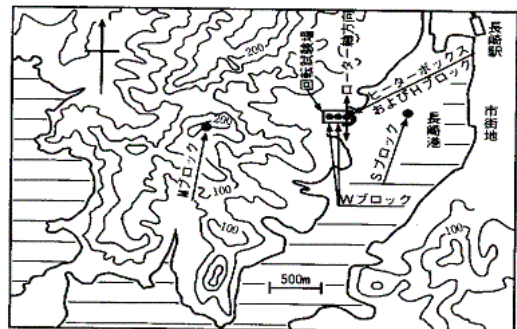
図3 飛散したロータの落下地点
